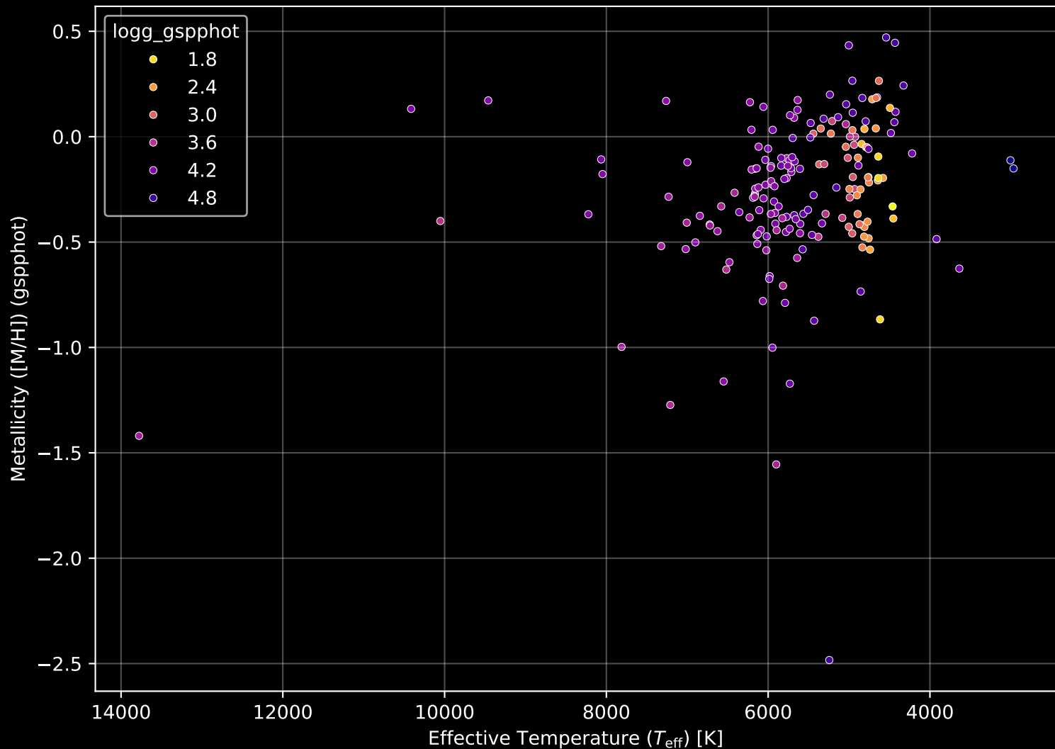
APOGEE DR17 Field: [CVZ_FILL01_btx] Stellar Population Parameters (n= 185)
